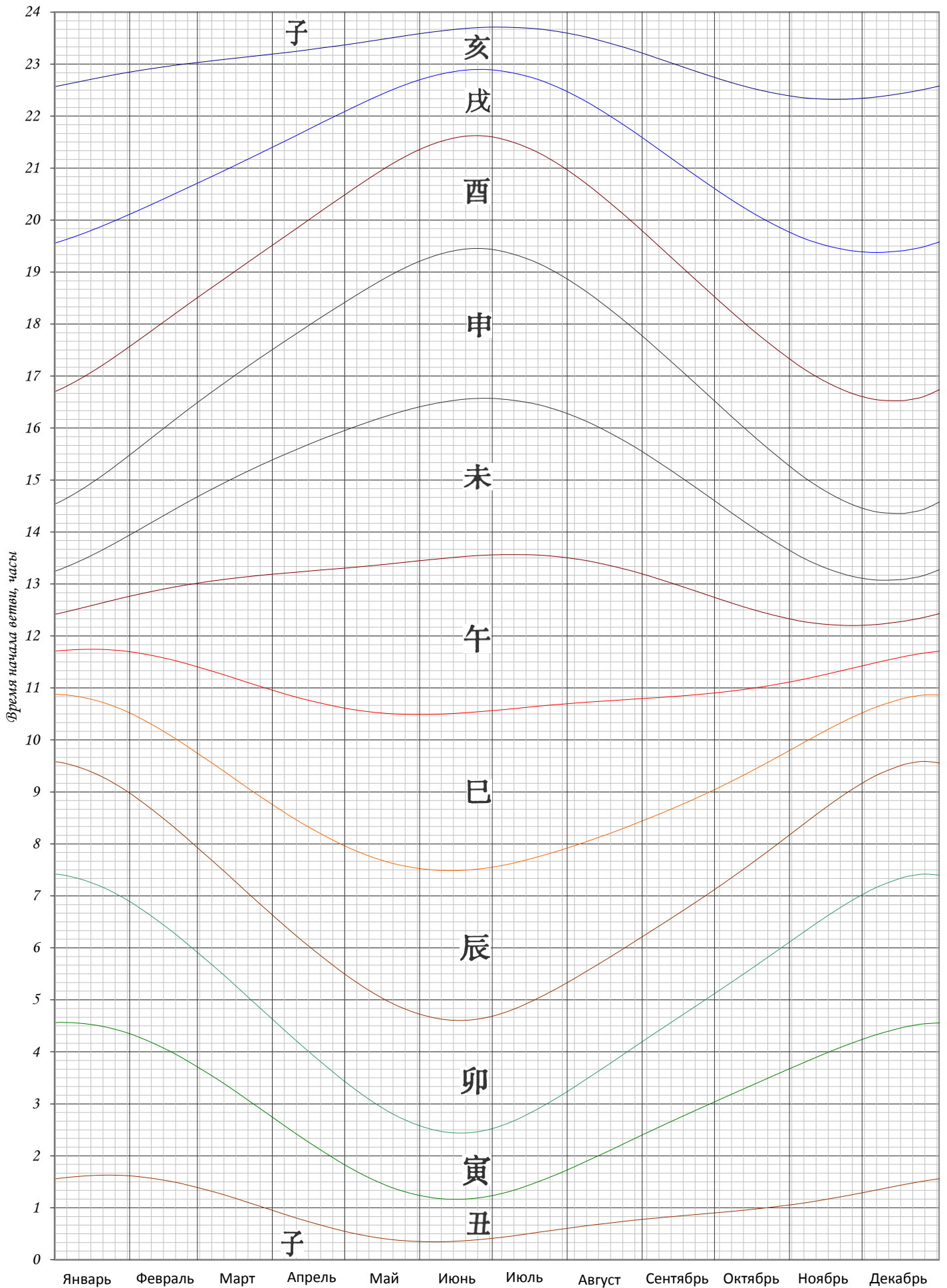
График ветвей часа для широты Москвы
